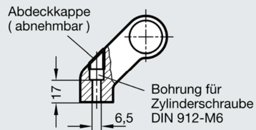
Form B Montage von der Bedienungsseite (nur für d_1 = 28 )
