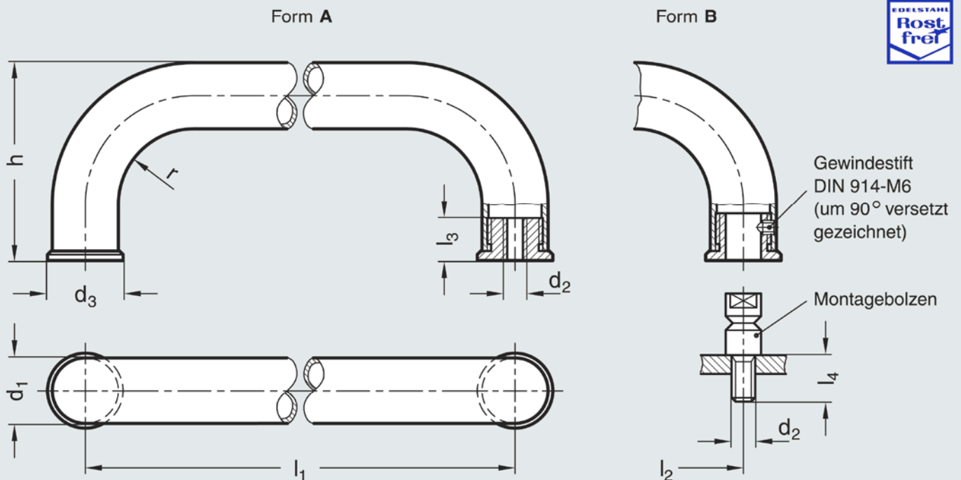
Form A Montage von der Rückseite (Gewinde-Sackloch)
